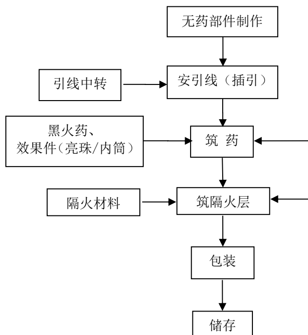
图 2.4-5 礼花类（小礼花/球形）产品生产工艺流程图
