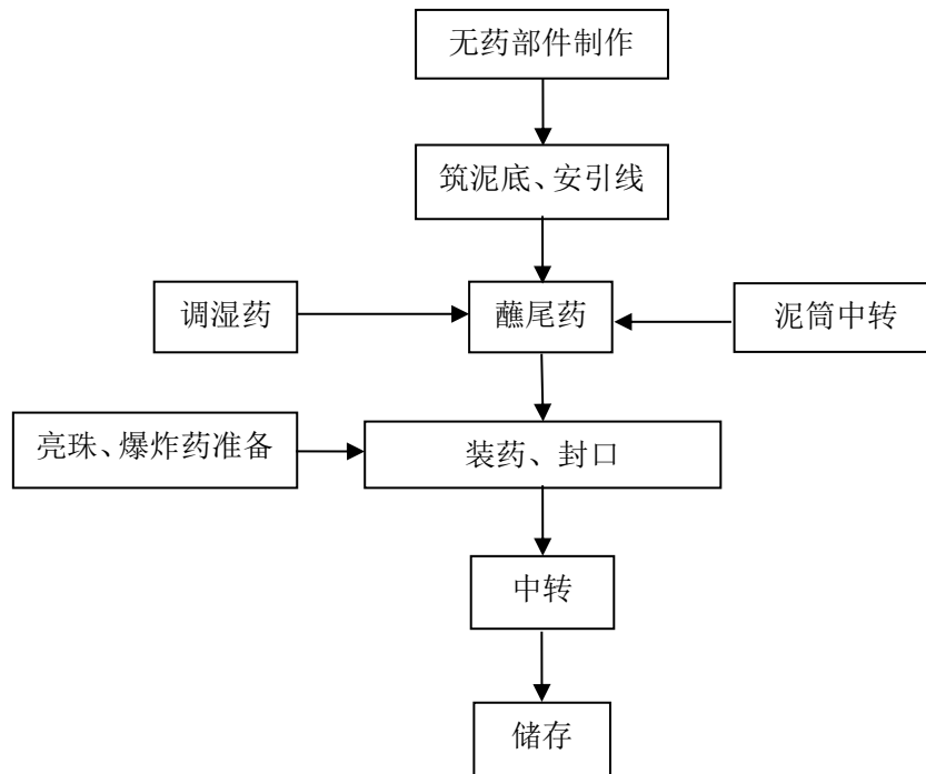
图 2.4-1 效果件内筒生产工艺流程图
