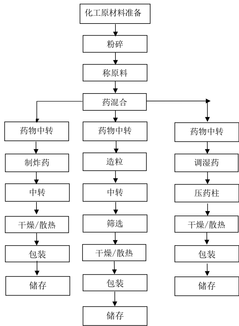
图 2. 4-2 药物裸药效果件（炸药、亮珠、药柱）生产工艺流程图
