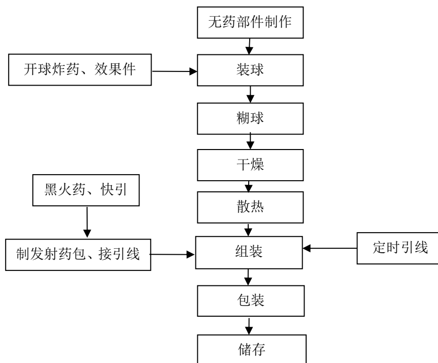
图 2.4-5 礼花类（小礼花/球形）产品生产工艺流程图
